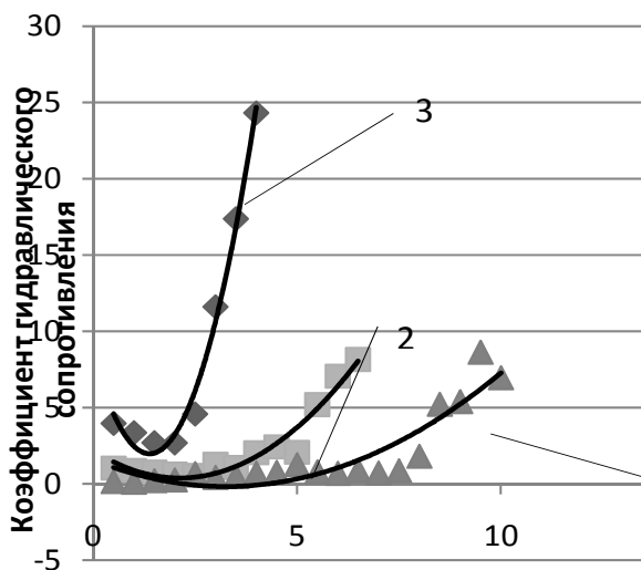
Рис. 3 – Зависимость гидравлического сопротивления от продолжительности перекачки нефти с содержанием воды 70% масс.: 1 – при давлении 2 кгс/см 2 ; 2 – при давлении 4 кгс/см 2 ; 3 – при давлении 6 кгс/см 2
