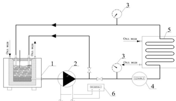
Рис. 1 – Схема установки по определению эффекта Томса: 1 – емкость, 2 – насос, 3 – манометры, 4 – расходомер, 5 – змеевик, 6 – электросчетчик
