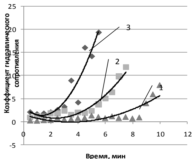
Рис. 4 – Зависимость гидравлического сопротивления от продолжительности перекачки нефти с содержанием воды 70% масс.: 1 – при давлении 2 кгс/см 2 ; 2 – при давлении 4 кгс/см 2 ; 3 – при давлении 6 кгс/см 2
