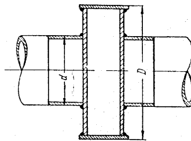
Рис. 2 – Схема линзового компенсатора с плоскими кольцевыми вставками.
