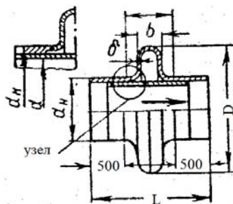
Рис. 1 – Схема линзового компенсатора с торообразными вставками
