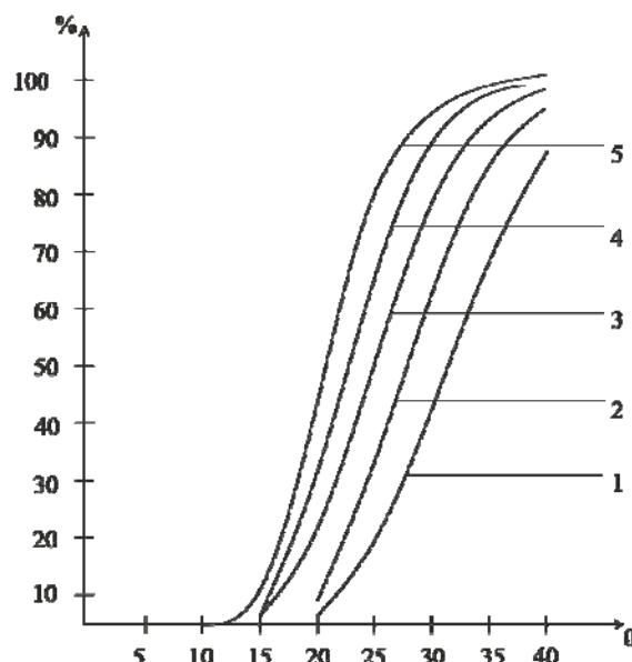
Рис. 1 - Граф работы системы при различных \lambda
