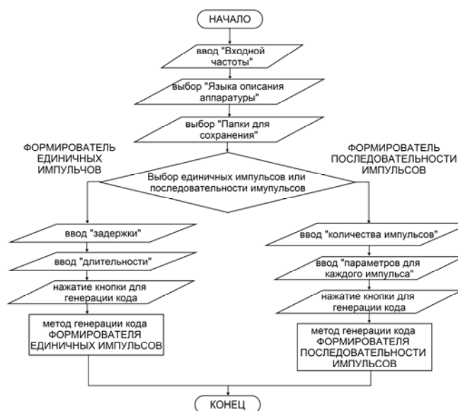
Рис. 2 – Обобщенный алгоритм работы приложения параметризованного автогенератора программного кода формирователя импульсов на языках описания аппаратуры Verilog/VHDL
