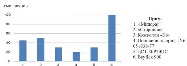
Рис. 5 - Сравнительные показатели сопротивления многократному изгибу полимерных подошвенных материалов
