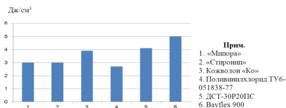
Рис. 4 - Сравнительные показатели сопротивления истиранию полимерных подошвенных материалов
