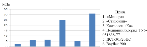
Рис. 2 - Сравнительные показатели прочности полимерных подошвенных материалов
