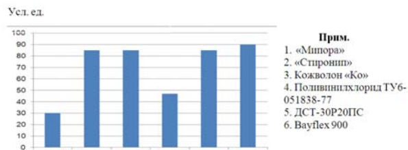
Рис. 3 - Сравнительные показатели твердости полимерных подошвенных материалов
