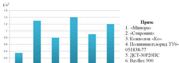
Рис. 1 - Сравнительные показатели плотности полимерных подошвенных материалов
