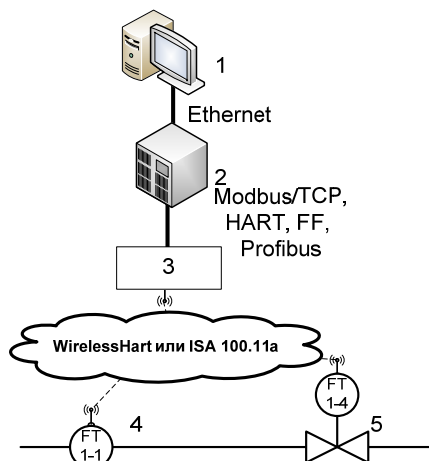
Рис. 1 - Организация системы управления с использованием беспроводных сетей: 1 - станция оператора технолога или инженерная станция, 2 - контроллер системы управления, 3 - шлюз беспроводной сети, 4 - беспроводные датчики, 5 - беспроводные исполнительные механизмы
