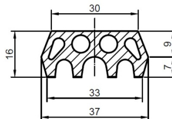
Рис. 1 – Поперечное сечение резиновой уплотнительной прокладки
