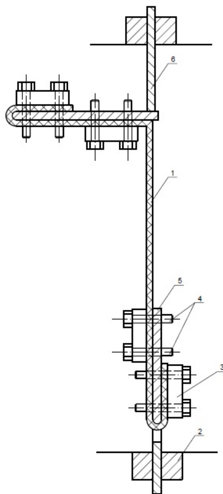
Рис. 3 – Схема крепления уплотнительной прокладки при определении прочности углового соединения.
