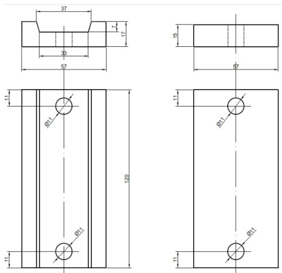
Рис. 4 – Струбцины для обжатия уплотнительных прокладок
