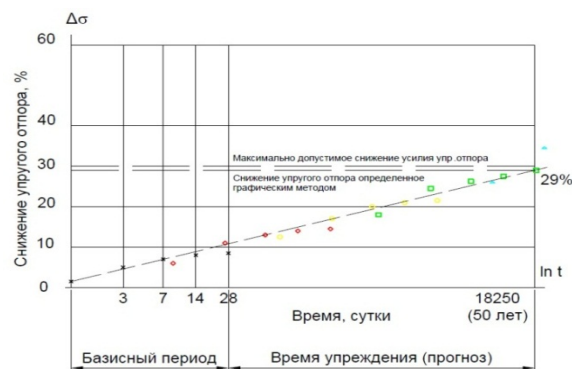
Рис. 6 – График прогноза изменения упругого отпора
