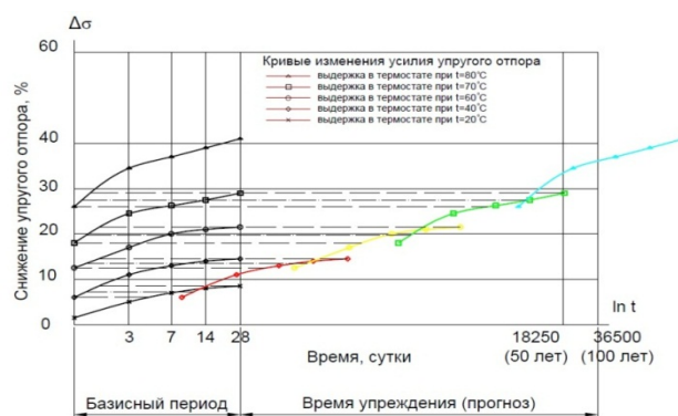
Рис. 5 – Графический способ прогнозирования изменения упругого отпора
