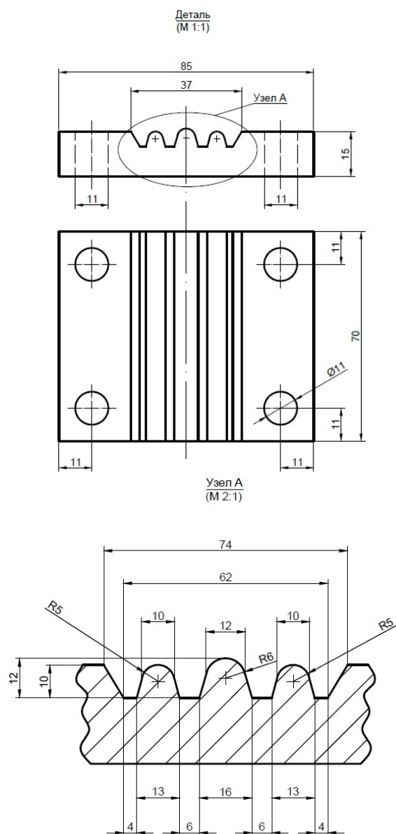
Рис. 2 – Приспособление для захвата резины при определении относительного удлинения и прочности основного сечения.
